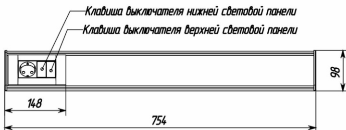
СВЕТИЛЬНИК СНС-16/40-Л (ЛЕВОСТОРОННЯЯ МОДИФИКАЦИЯ)
