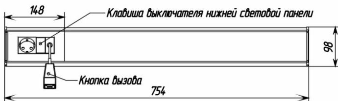
СВЕТИЛЬНИК СНС-16/40-Л (ЛЕВОСТОРОННЯЯ МОДИФИКАЦИЯ)
